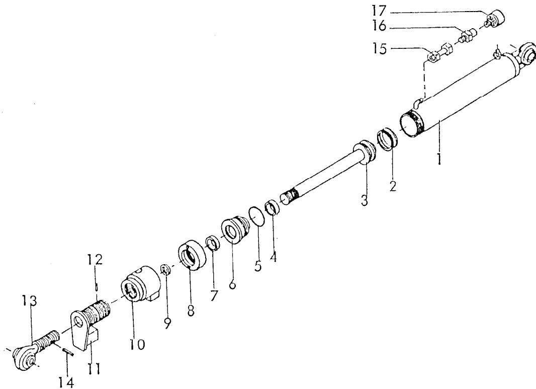
Gerätetyp: Hydr. Zylinder \varnothing 80 -einfachwirkend- für XF-450, 600 ( Deichsel )
