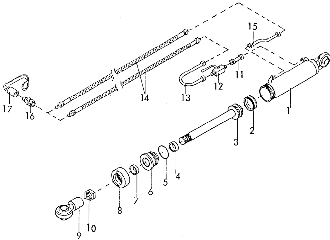
Gerätetyp: Zylinder \varnothing 65 -doppeltw.- für hydr. Schwenkeinrichtung FPL-215,270 Br.1
