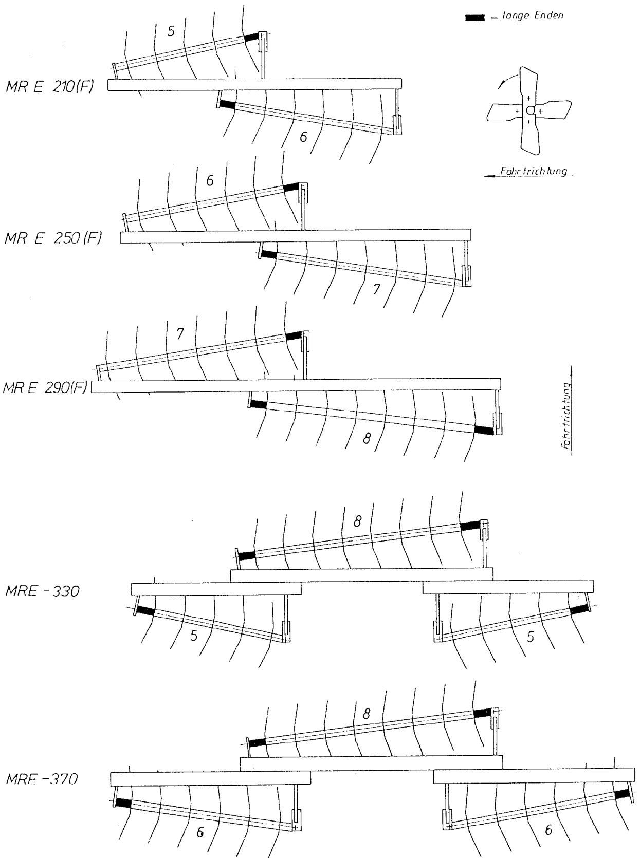
Messerrollegge MRE 210,250,290,330,370 -einreihig- Messer und Messerwellenanordnung
