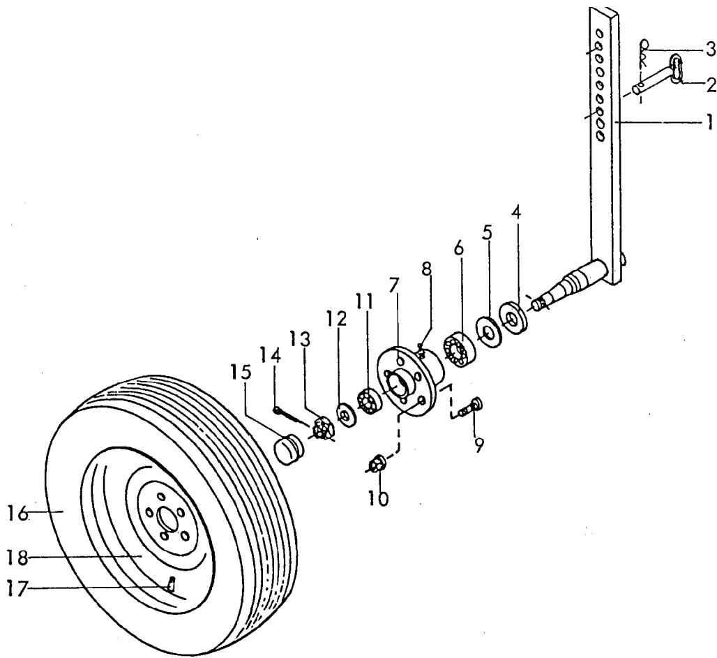
Gerätetyp: Stützräder für RKZ 500,560,610,660,840 D
