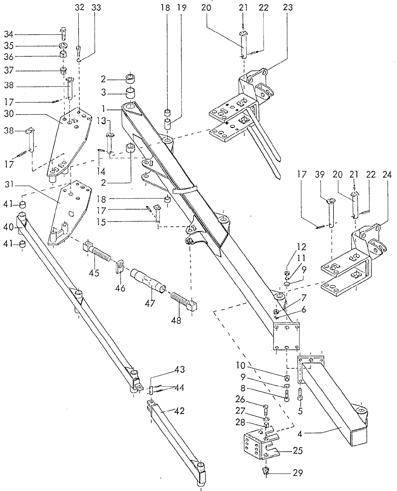
4763 Supertube-Vari-Avant 160 CD, MCD Baureihe 2 06.88
