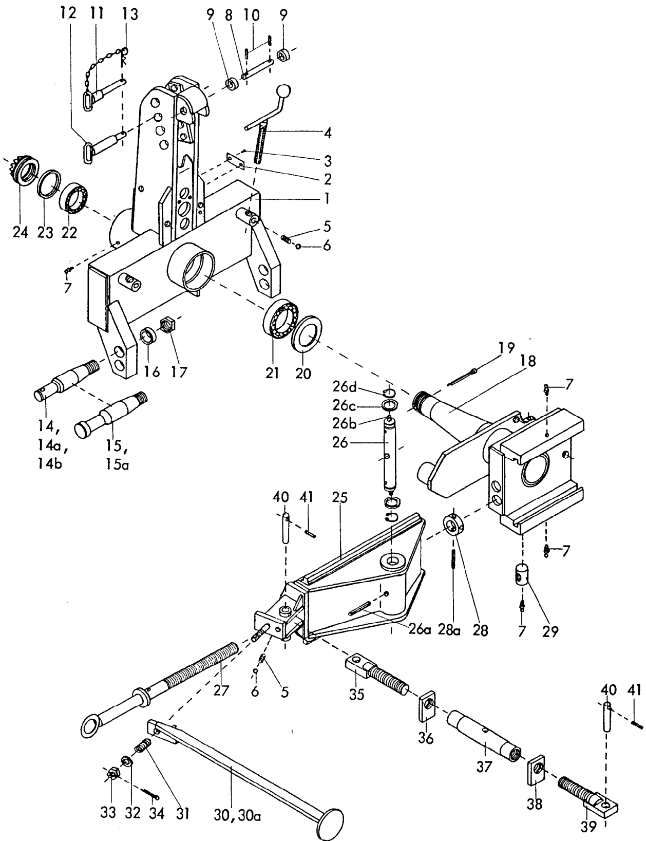
4723 LMGE(D), Supertaube LGE(D), GE(D), MGE(D), KGE(D) Baureihe 5 Supertaube-Avant LGE(D), GE(D) Baureihe 4 12.83
