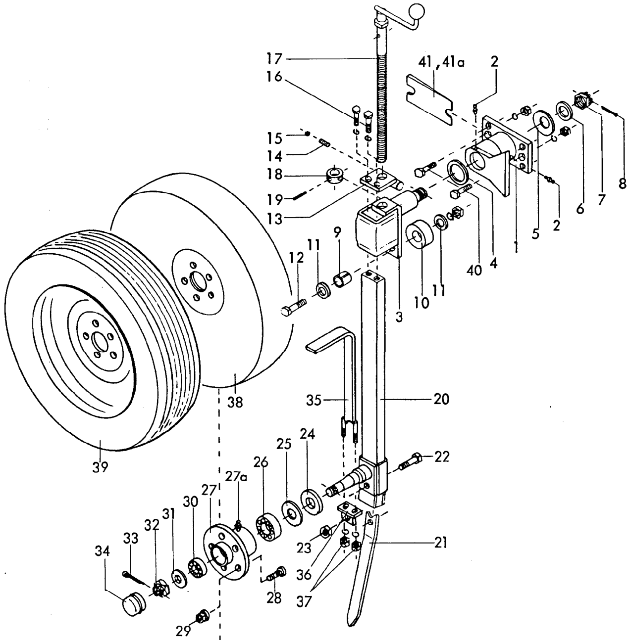
Gerätetyp: Pendelstützrad PS 600/130, PS 13
