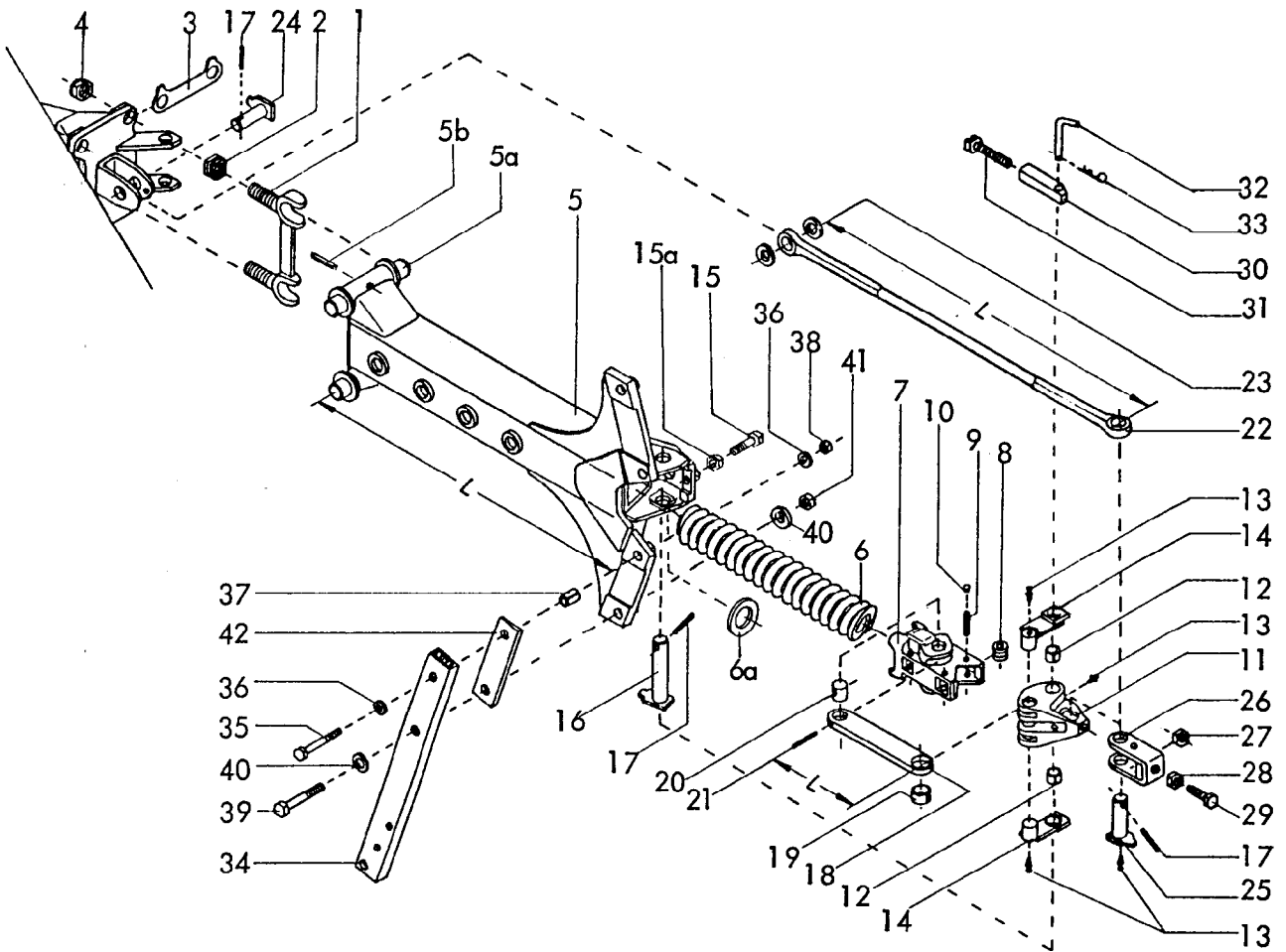
Gerätetyp: Supertaube-Avant GE(D) Baureihe 4
