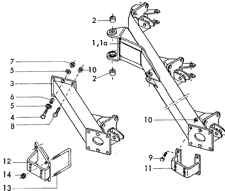
Gerätetyp: Supertaube-Avant LGE(D), LMGE(D), GE(D) Baureihe 4
