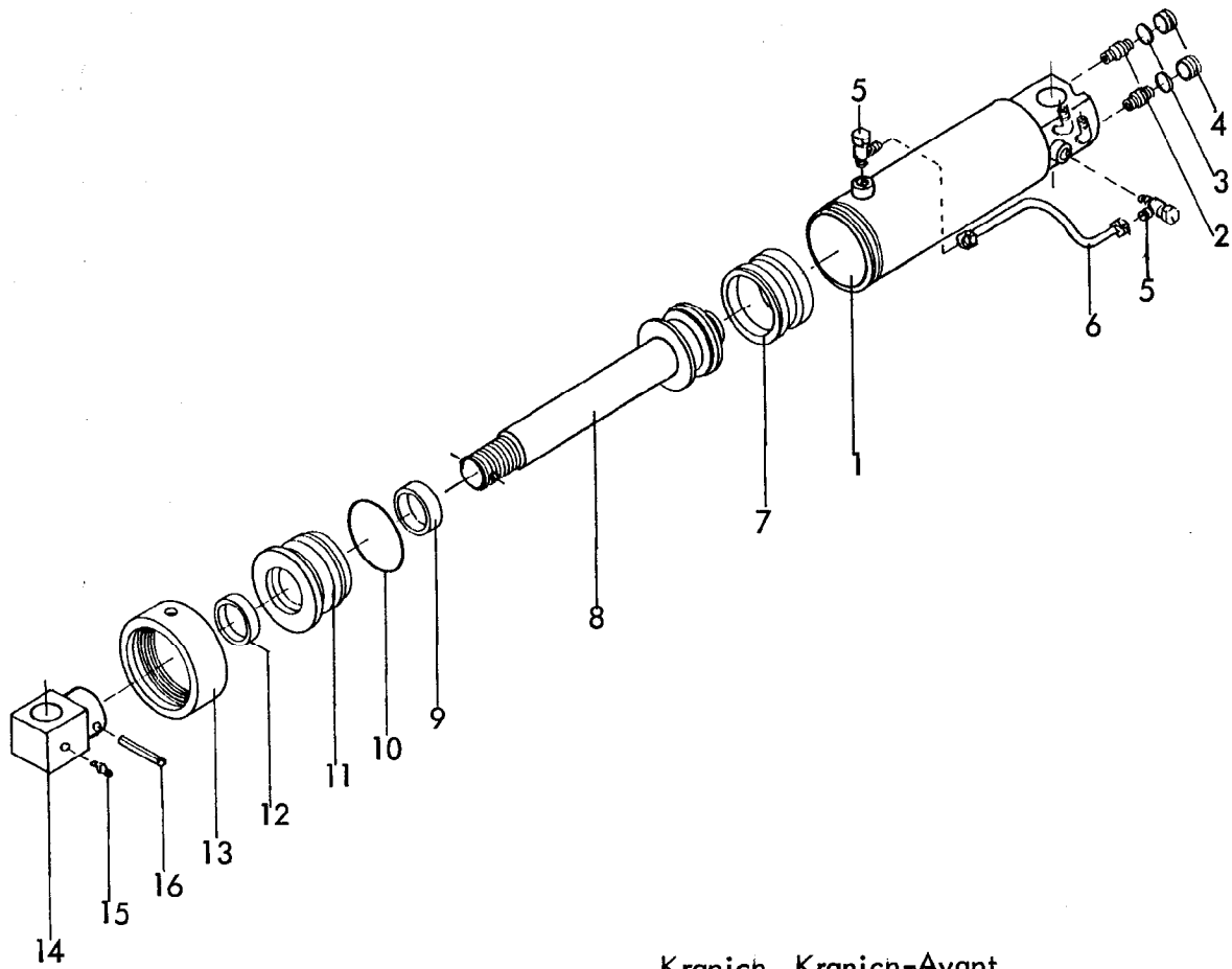
Kranich, Kranich-Avant
