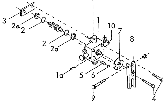
4766 / 4767 Kranich, Kranich-Avant 180 A, AS Baureihe 1, 2, 3 -Hydraulik Vordere Abdeckplatte- 04.89
