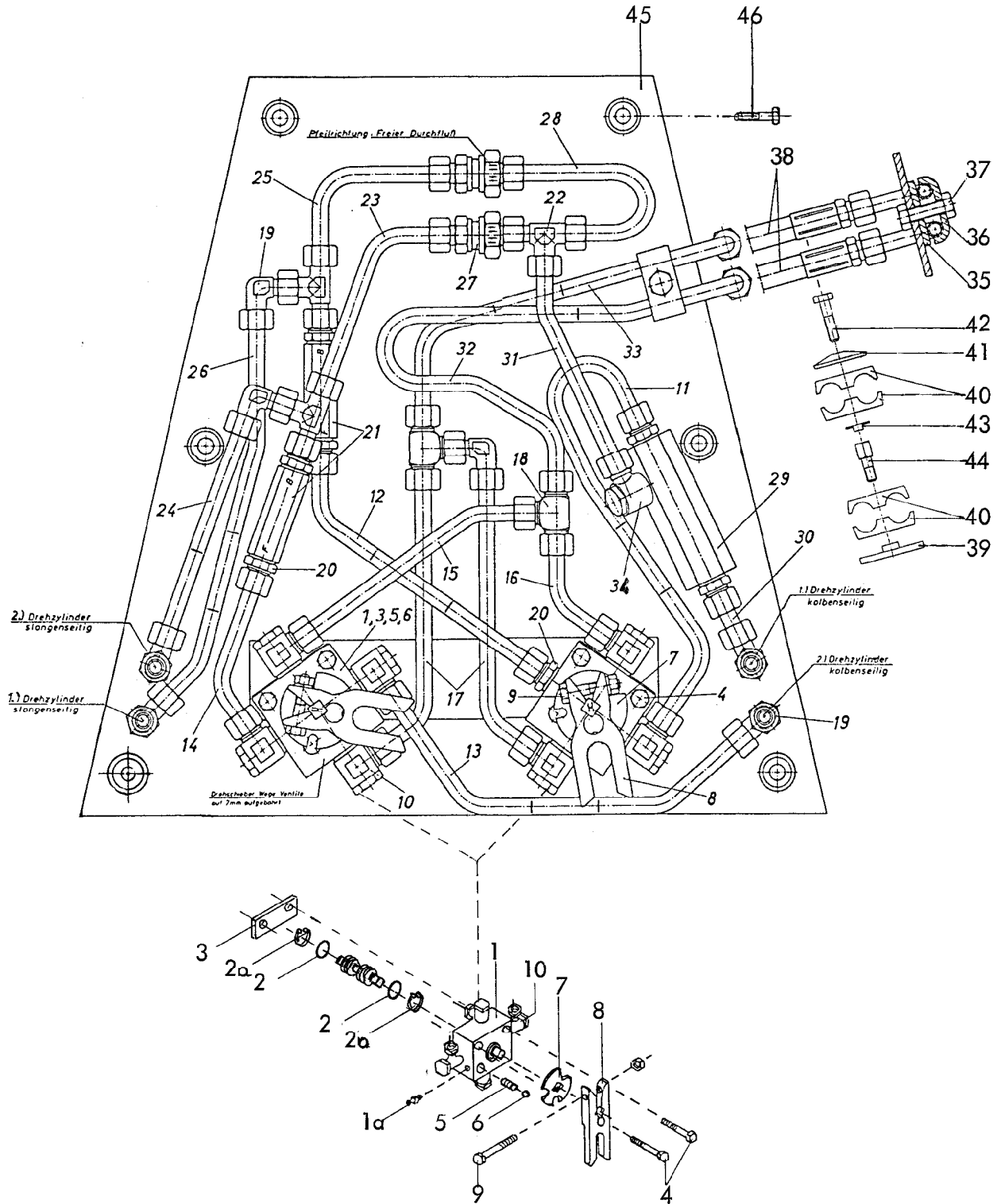
4754 Kranich, Kranich-Avant 160 A Baureihe 3 -Hydraulik Vordere Abdeckplatte- 03.89
