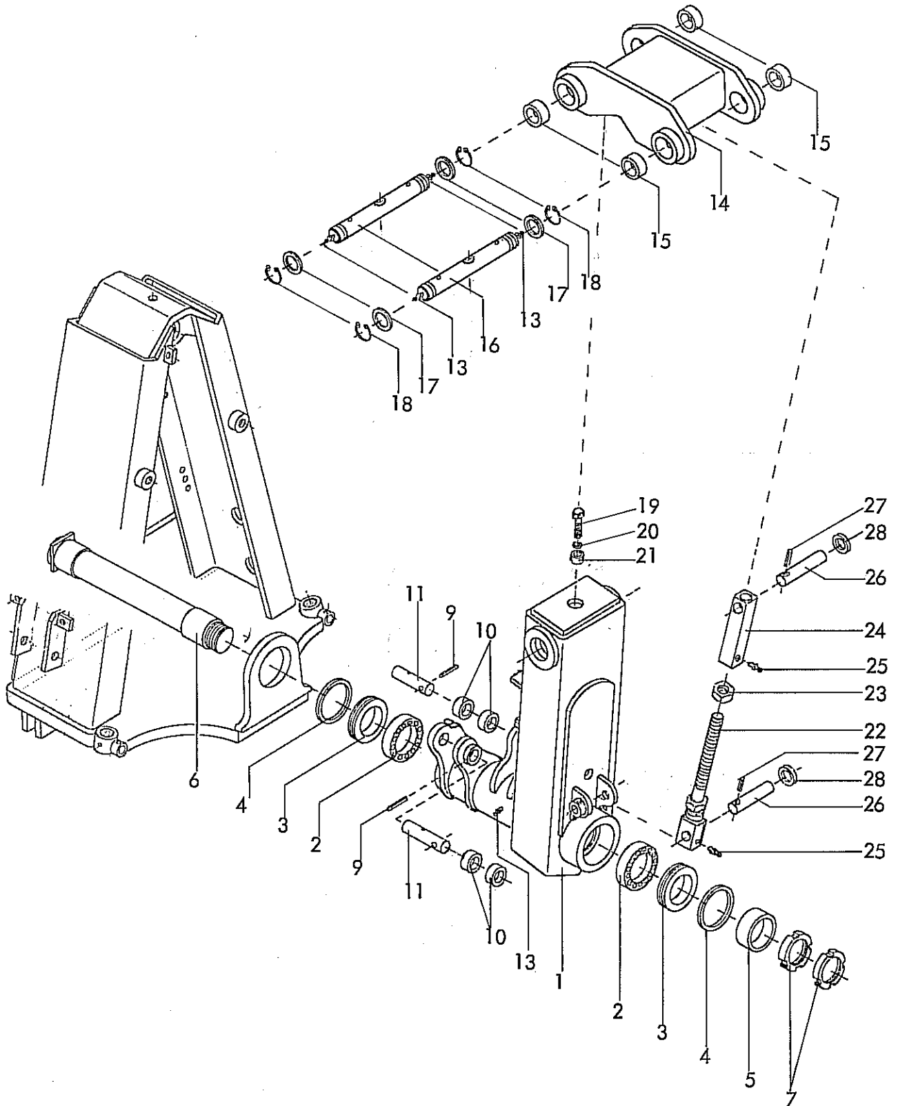
4754 Kranich, Kranich-Avant 160 A Baureihe 3 -Wendearm- 03.89
