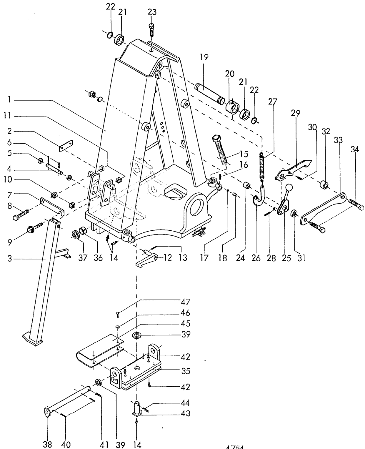
4754 Kranich, Kranich-Avant 160 A Baureihe 3 -Traverse- 03.89
