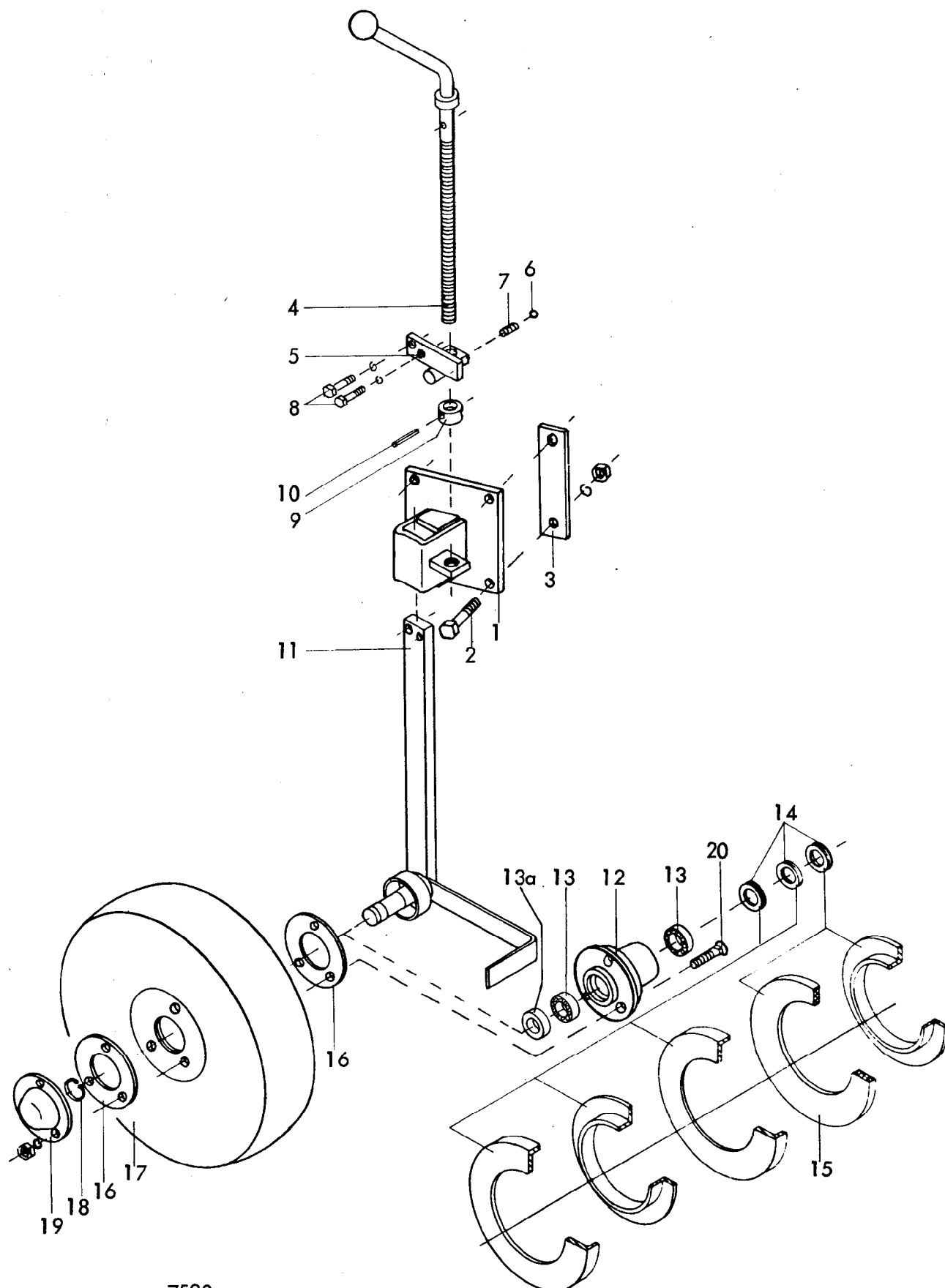
7520 Tastrad S 500/120 für Pirol Br. A , B 09.85
