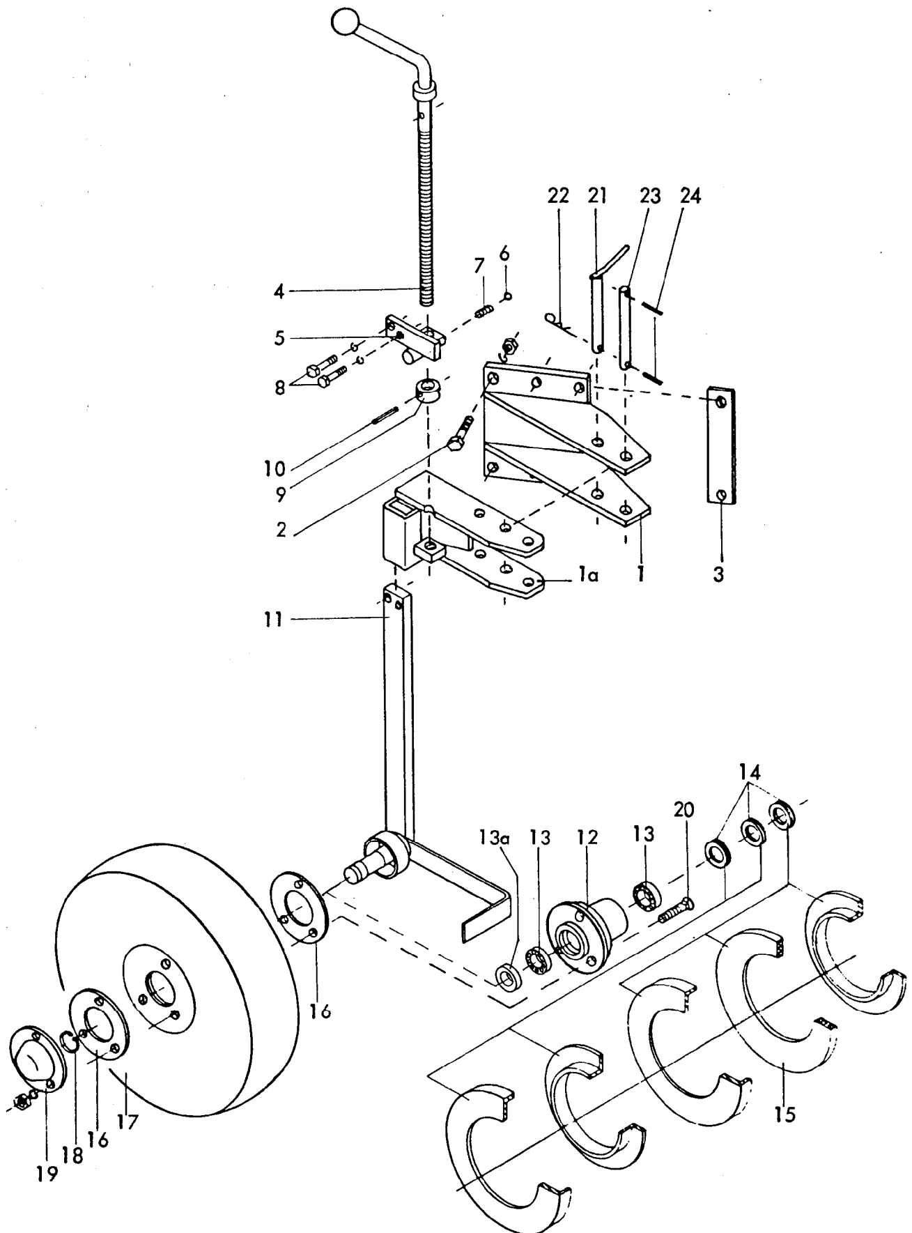
7520 Schwenkbares Tastrad SE 500/120 für Pirol Br. A , B 09.85
