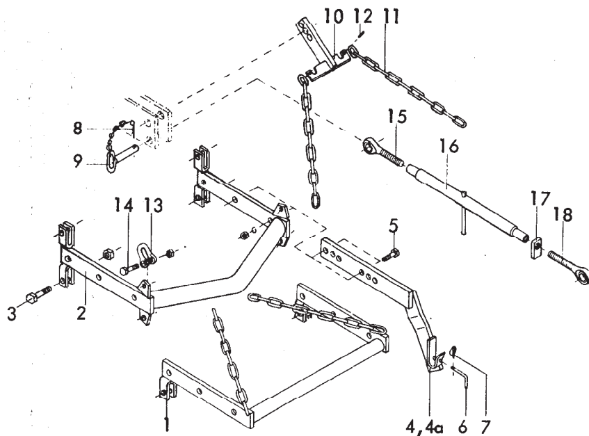
Gerätetyp: EMKE, WMKE -Dreipunktgestänge für Anbaugeräte-
