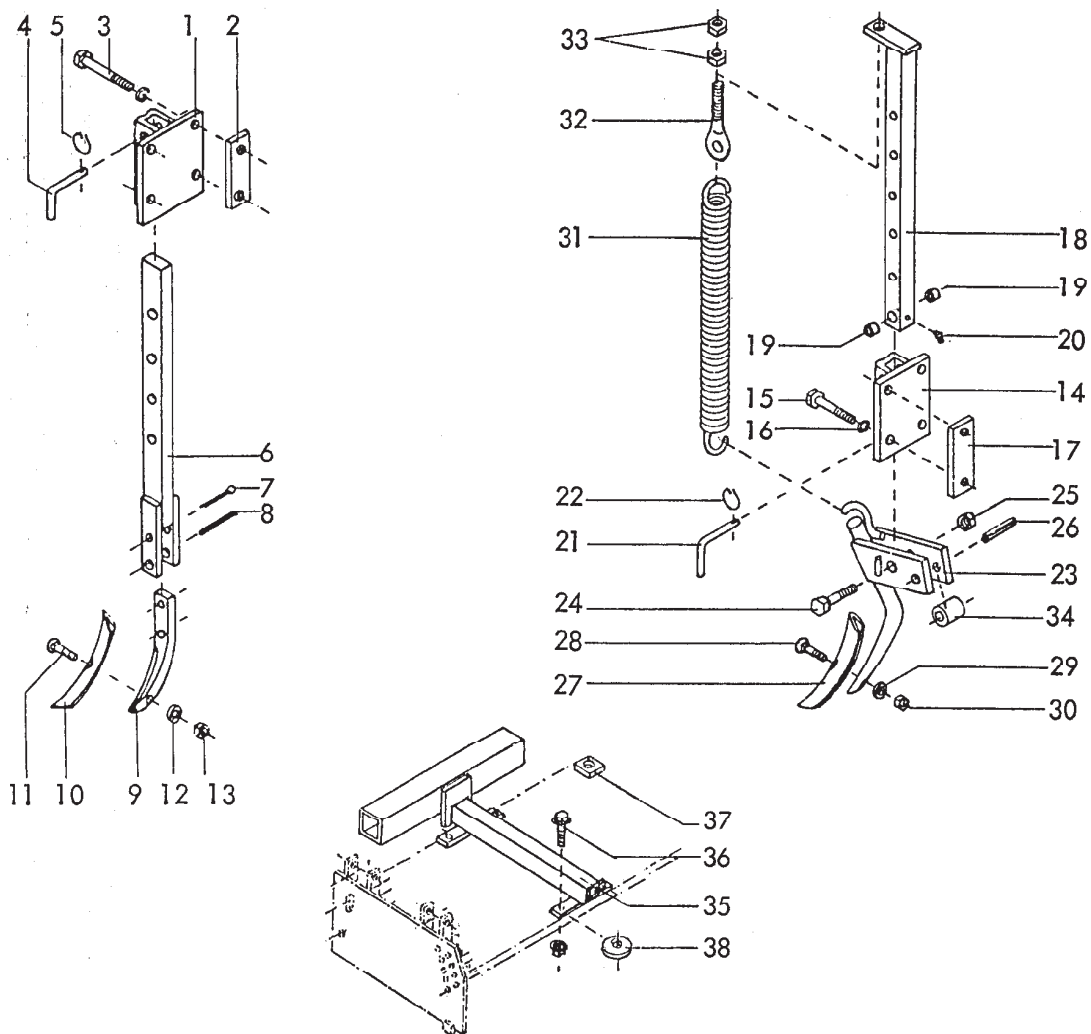
Gerätetyp: Radspurlockerer starr / gefedert für EMKE, WMKE 200,250,300
