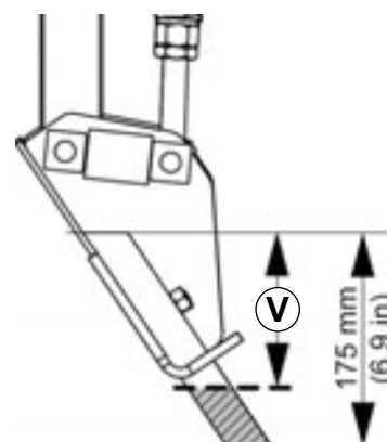
Fig. 97; Train denté - Dentées, seuil d'usure
