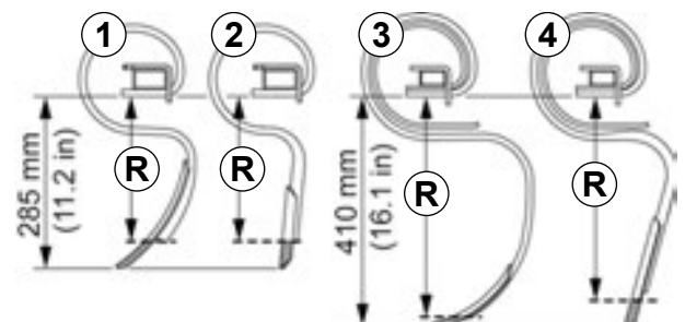
Fig. 91; Seuil d'usure des socs
