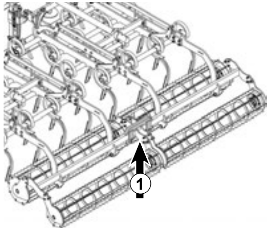
Fig. 109; Sturmvogel 3001 L
