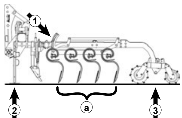
Fig. 92; Levage des dents
