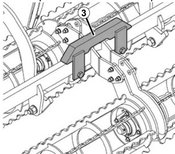
Fig. 30; Composant de sécurité - Raccord de rouleau pour dents d'émission à doubles pointes
