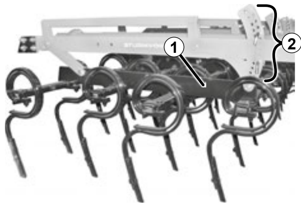
Fig. 60; Réglage de la position de travail
